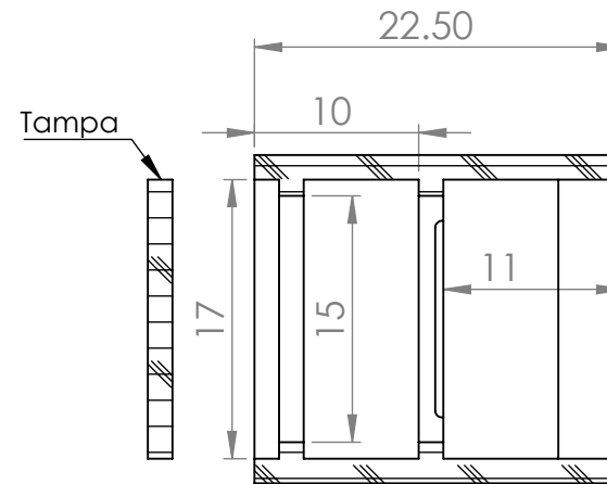
SEÇÃO A-A
